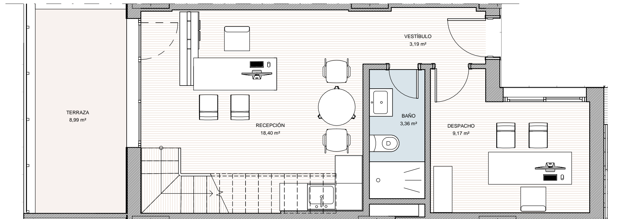
PLANTA BAJA
