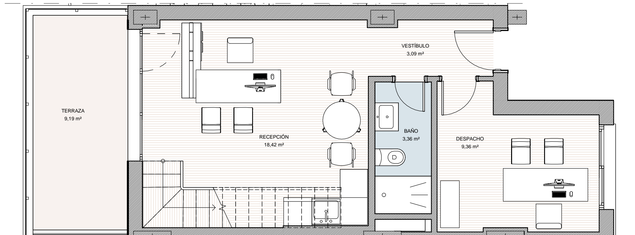
PLANTA BAJA
