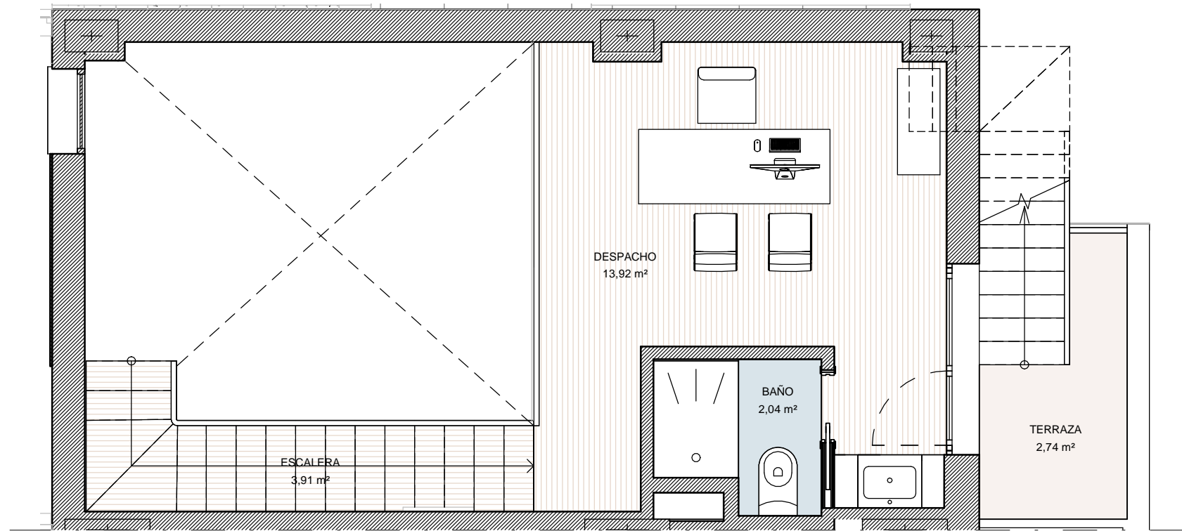
PLANTA PRIMERA
