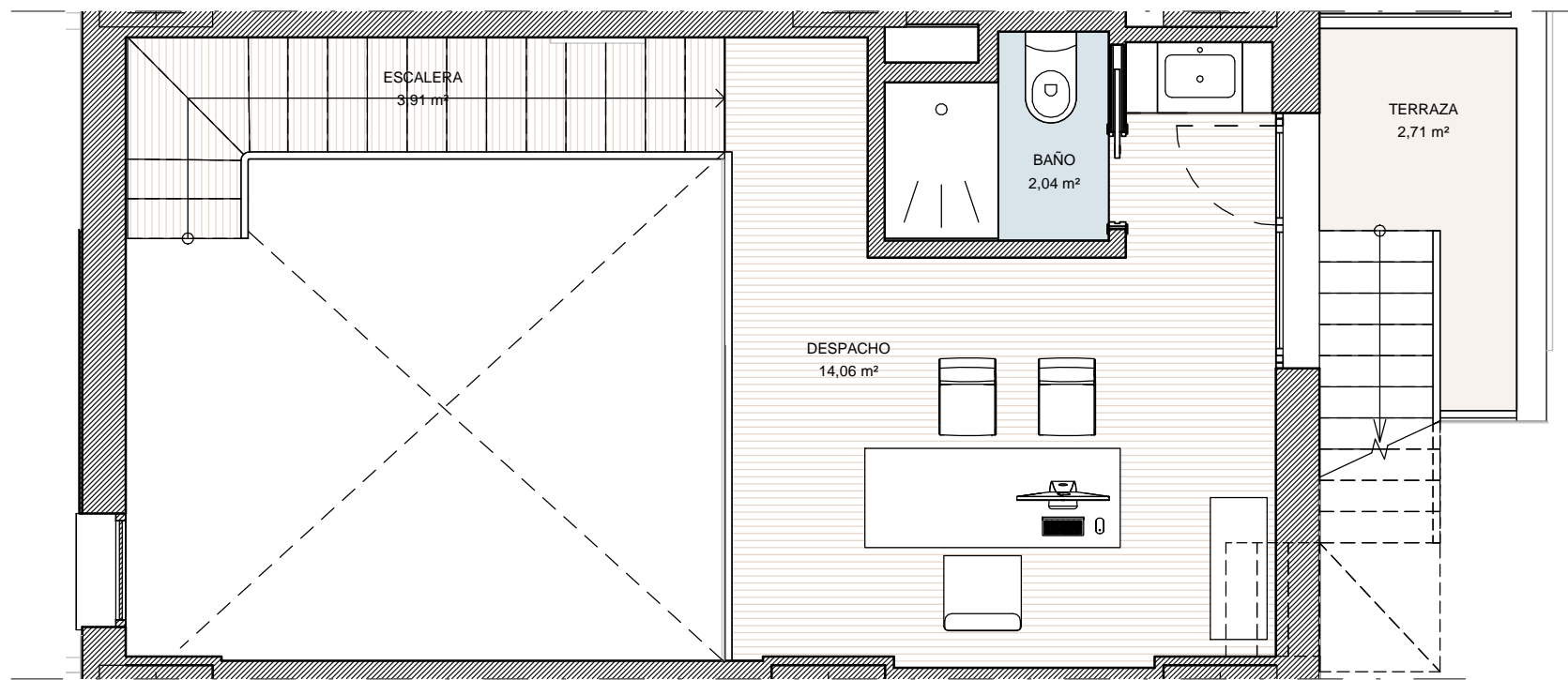
PLANTA PRIMERA
