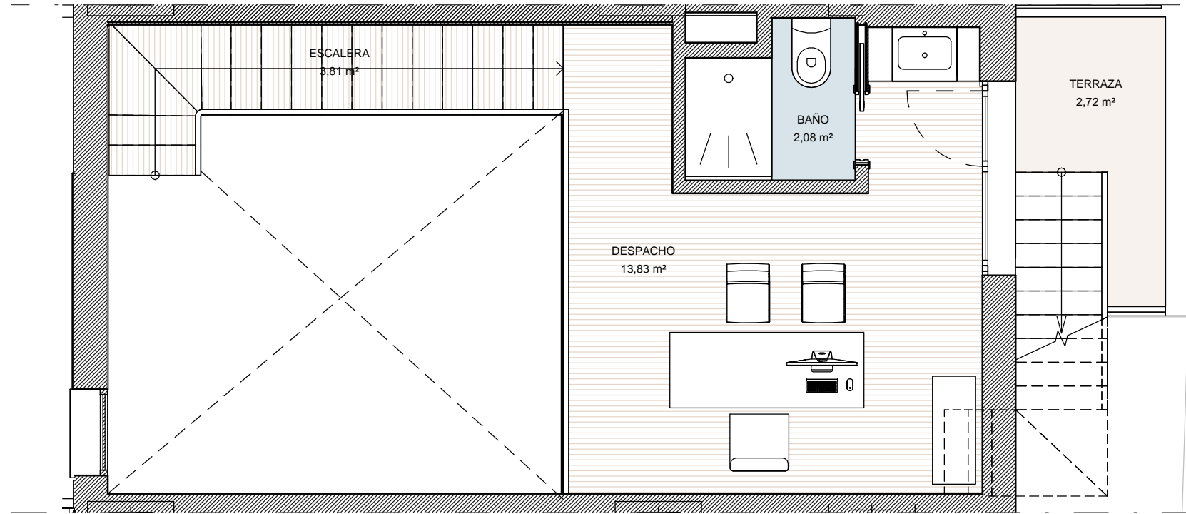
PLANTA PRIMERA
