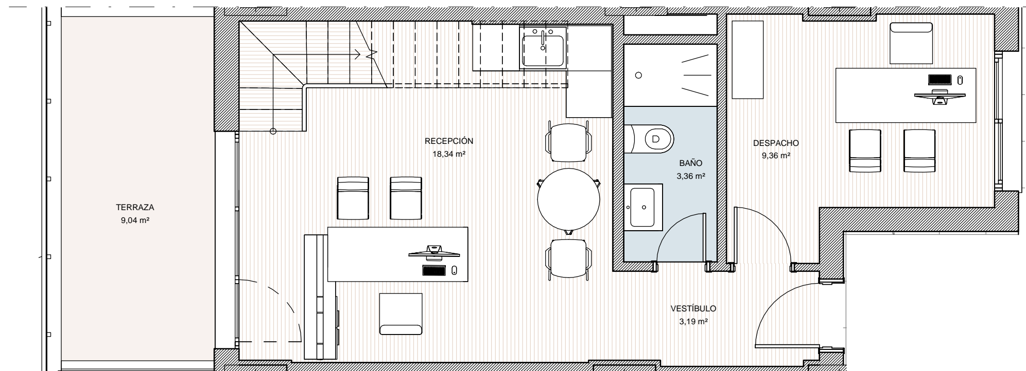
PLANTA BAJA
